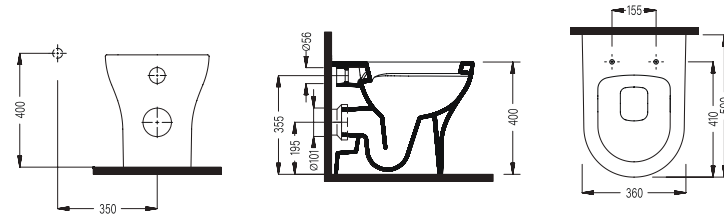
ROOT BTW WC PAN 50 CM WITHOUT BIDET FUNCTION COOL WHITE EXT. ROKK05001VPOW5SZ0
